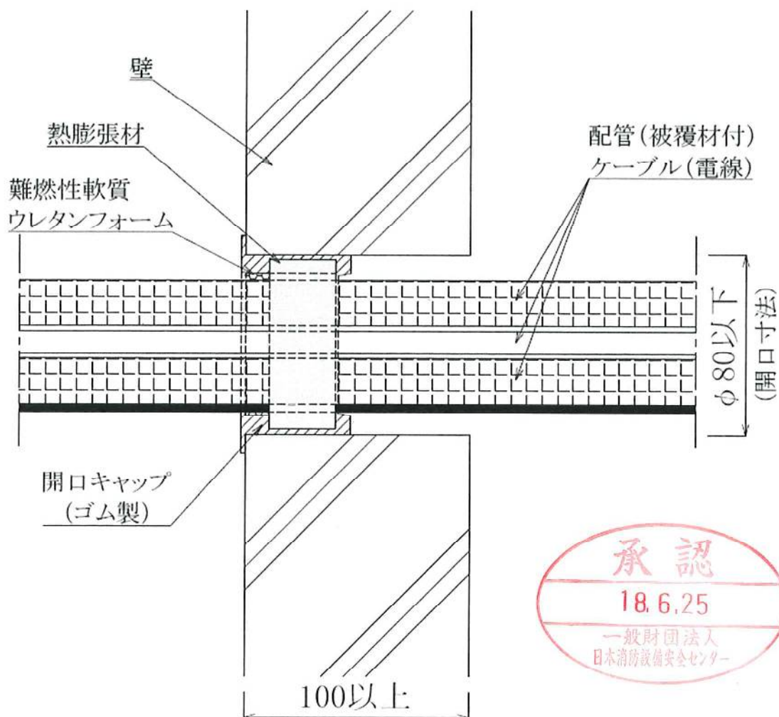
断面図</
